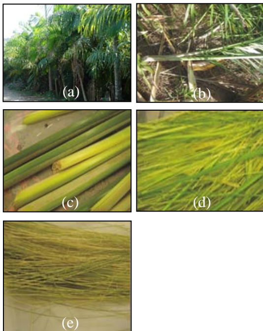
Figura 2: Imagens do processo de obtenção da fibra da pupunheira.
