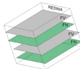
Figura 9: Modelo esquemático da disposição das fibras/tramas para a confecção dos corpos de prova.
