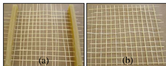
Figura 3: Fibras tramadas em suporte de elastômero de poliuretana e ajustadas com espaçamento de 1cm.
