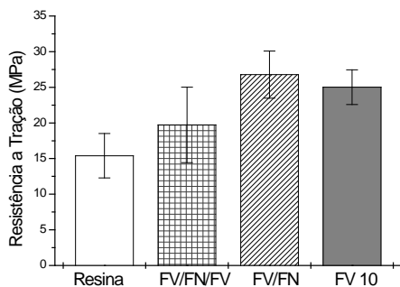
Figura 5: Comparativo de resistência a tração dos diferentes corpos de prova submetidos ao ensaio.
