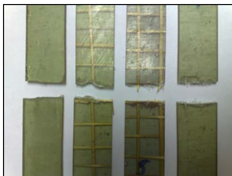
Figura 4: Corpos de prova submetidos ao ensaio de tração (a) resina, (b) 1FV/1FN, (c) 1FV/1FN/1FV e (d) FV.
