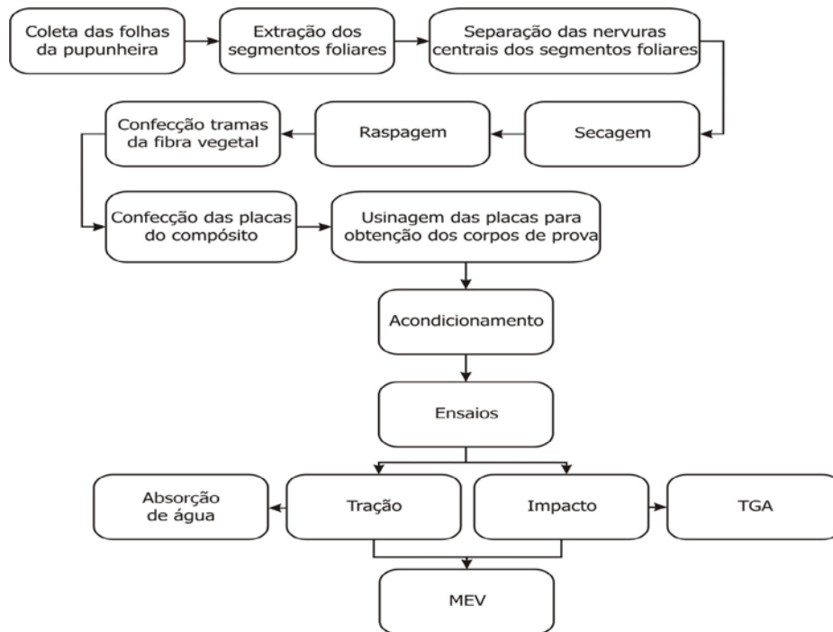
Figura 1: Fluxograma das etapas realizadas para a obtenção dos corpos de prova para realização dos ensaios.
