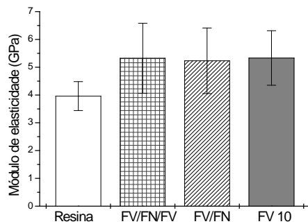
Figura 7: Comparativo do módulo de elasticidade dos diferentes corpos de prova submetidos a análise.
