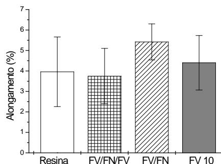
Figura 6: Comparativo do alongamento dos diferentes corpos de prova submetidos a análise.
