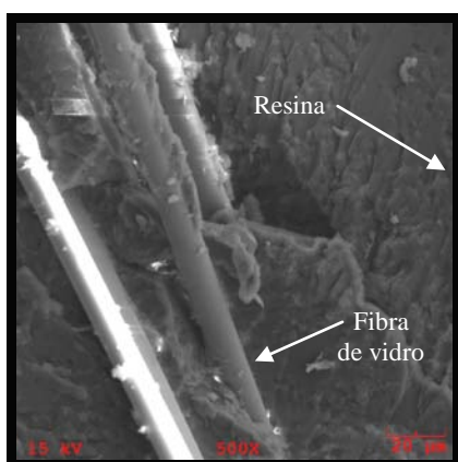
Figura 10: Micrografia da fratura do corpo de prova confeccionado com fibra de vidro submetido ao ensaio de tração.
