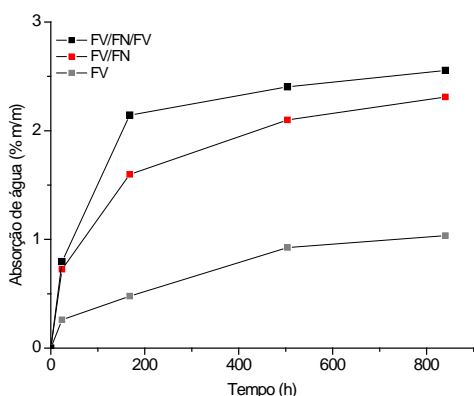
Figura 13: Percentual de absorção de água dos compósitos submetidos ao ensaio.
