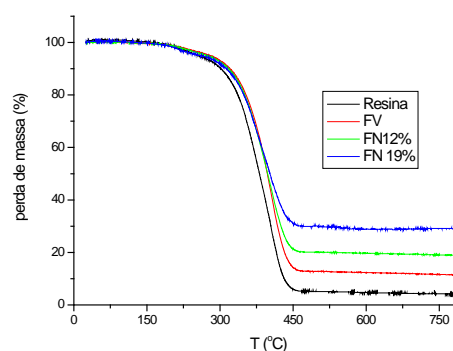
Figura 12: Comportamento térmico dos compósitos submetidos ao ensaio de degradação térmica.
