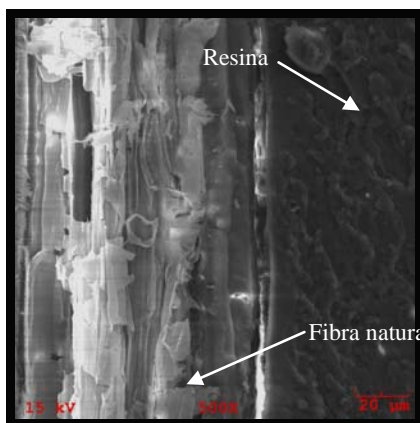
Figura 11: Corpo de prova confeccionado com uma manta de fibra de vidro e uma trama de fibra natural submetido ao ensaio de tração.
