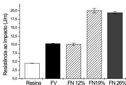
Figura 8: Comparativo de resistência ao impacto dos diferentes corpos de prova submetidos a análise.
